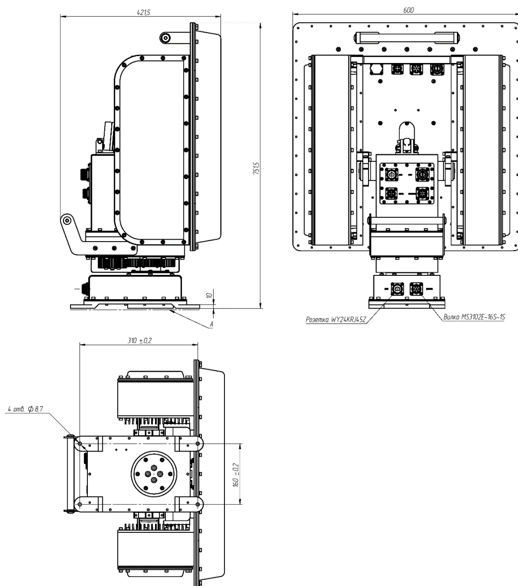
Рисунок 1 — Габаритные и установочные размеры Изделия (нулевое положение антенны в угломестной плоскости относительно установочной поверхности А)
